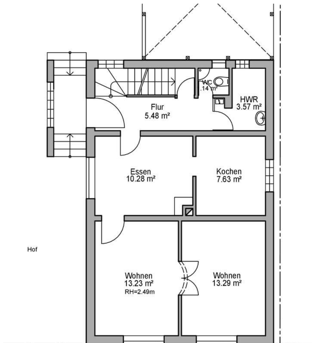
Grundriss Erdgeschoss
