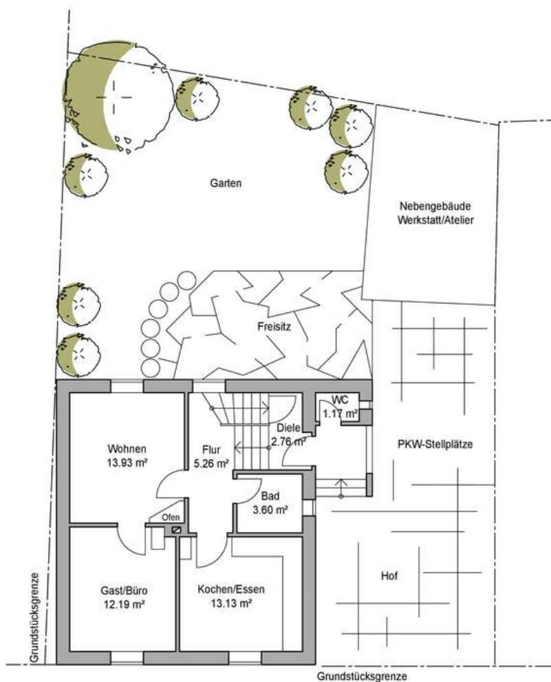
STRASSE Freiflächenplan o.M.
